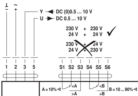
NRF24A-SZ-S2(-0) SRF24A-SZ-S2(-0)
