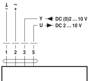
NRF24A-SR(-0) SRF24A-SR(-0)
