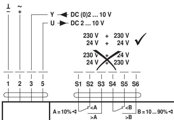
NRF24A-SR-S2(-0) SRF24A-SR-S2(-0)
