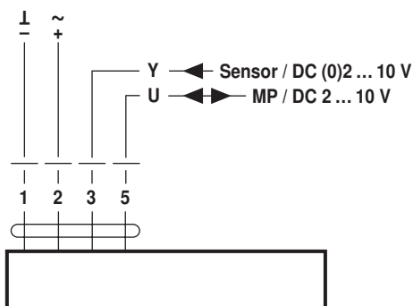
NRF24A-MP(-0) SRF24A-MP(-0)
